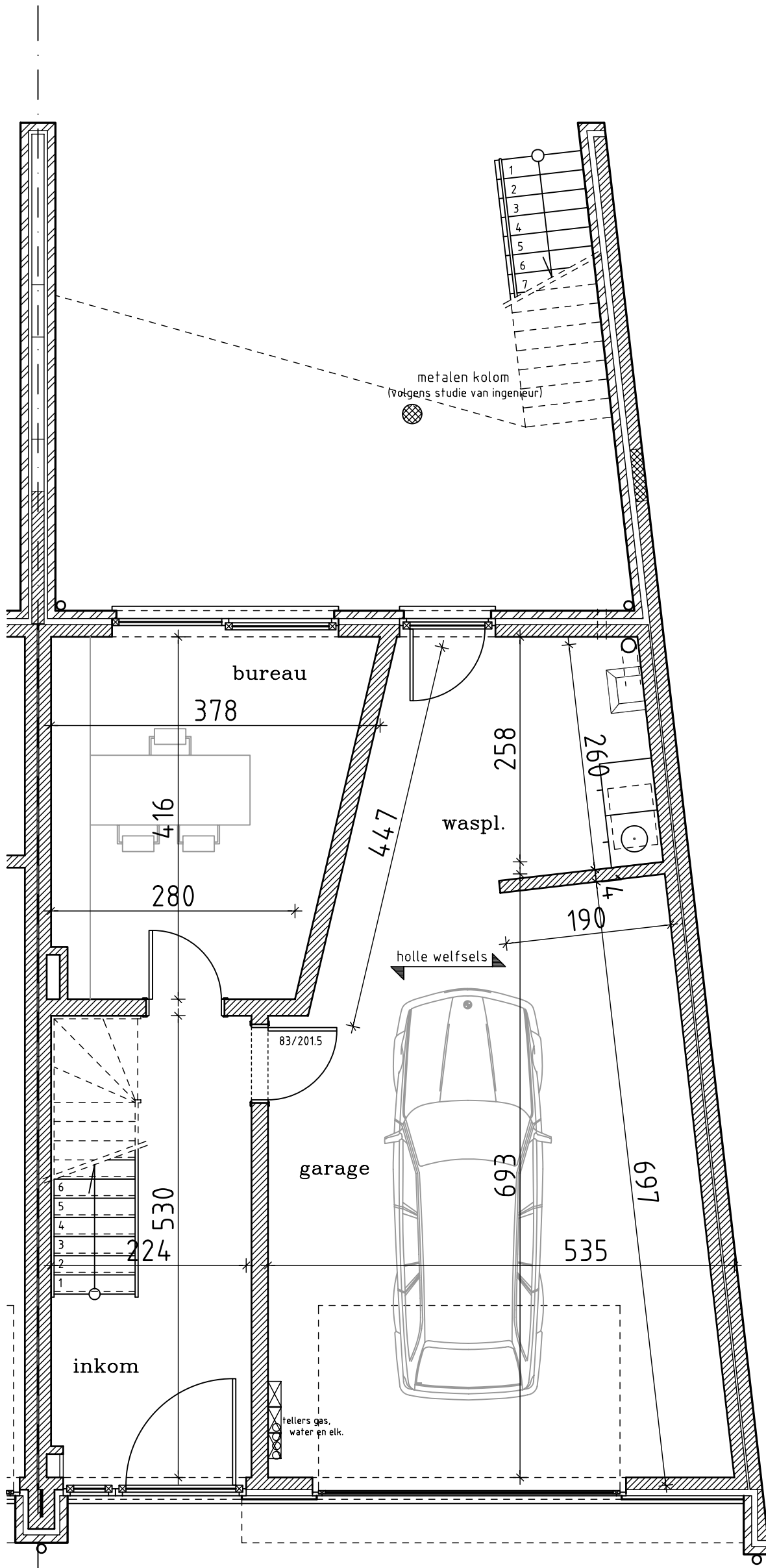
plan gelijkvloers
